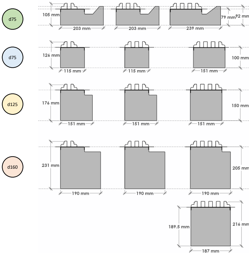
Plenum box + diffuser grill
